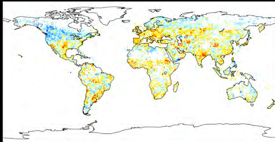
ODIAC CO2 vs TCR-2 NOx : 2011-2017
