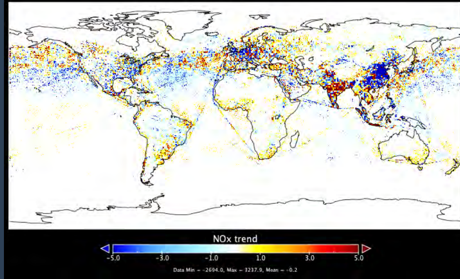
TCR-2 NO x trend : 2011-2017
