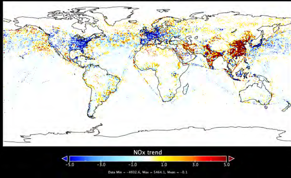
TCR-2 NO x trend : 2005-2010
