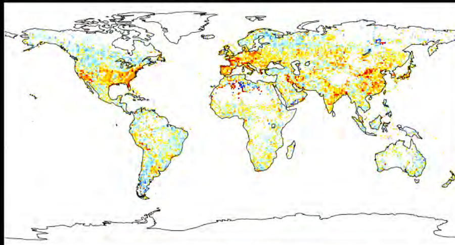
ODIAC CO2 vs TCR-2 NOx : 2005-2010
